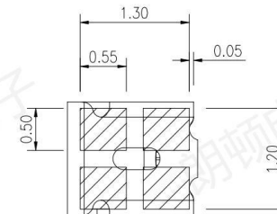
焊盘推荐尺寸
