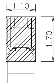
P.C.B焊盘尺寸 公差: \pm 0.05\text{MM}
